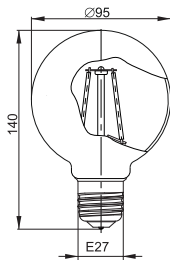
Рисунок 10 – Лампа LED-G95 серия 360° 6 Вт, 8 Вт цоколь E27
